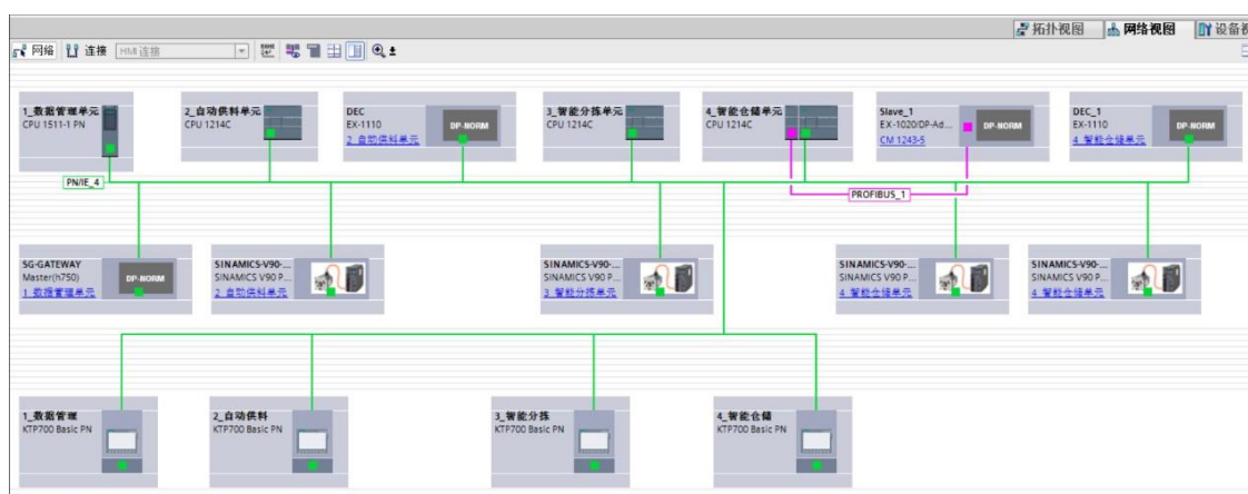
图3 系统组态截图（参考）
