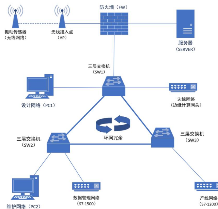
图 2 工业网络系统结构示意图
