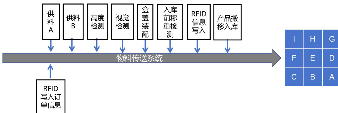
图 1 系统工艺流程示意图
